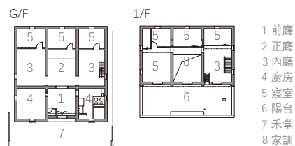
何氏大宅平面圖
