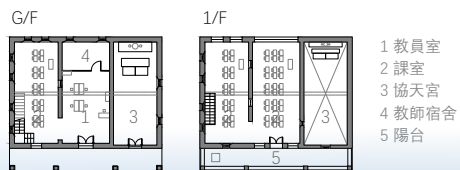
啟才學校平面圖
