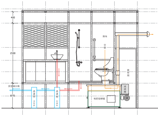
廁所處理模組功能圖
